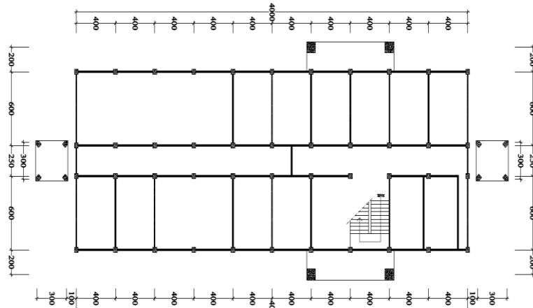
Gambar 5. 12 Denah Lantai 1 Kantor Bidang Ekonomi, Pembangunan dan Kesra Kampar
