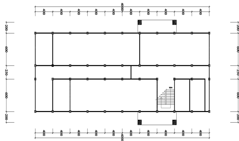
Gambar 5. 13 Denah Lantai 2 Kantor Bidang Ekonomi, Pembangunan dan Kesra Kampar
