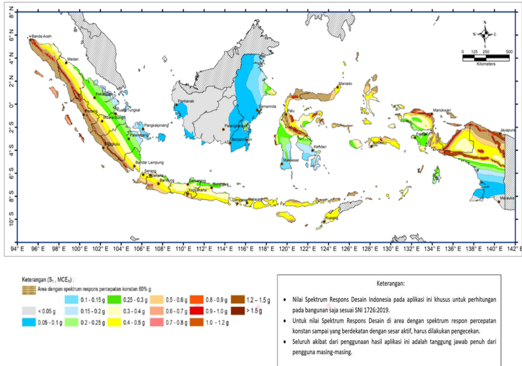
Gambar 3. 4 Akselerasi respon spektrum, S1 Sumber : (PUPR, 2021)
