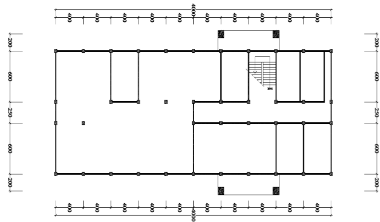
Gambar 5. 16 Denah Lantai 2 Kantor Tata Pemerintahan, Hukum, dan Politik Kampar
