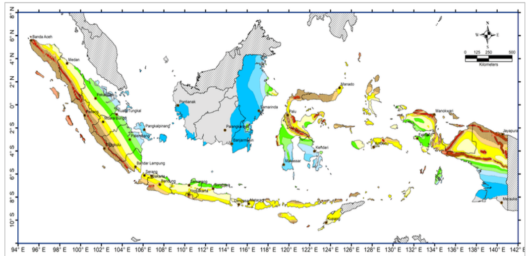
Gambar 5. 7 Akselerasi respon spektrum, S1 Sumber : (PUPR, 2021)
