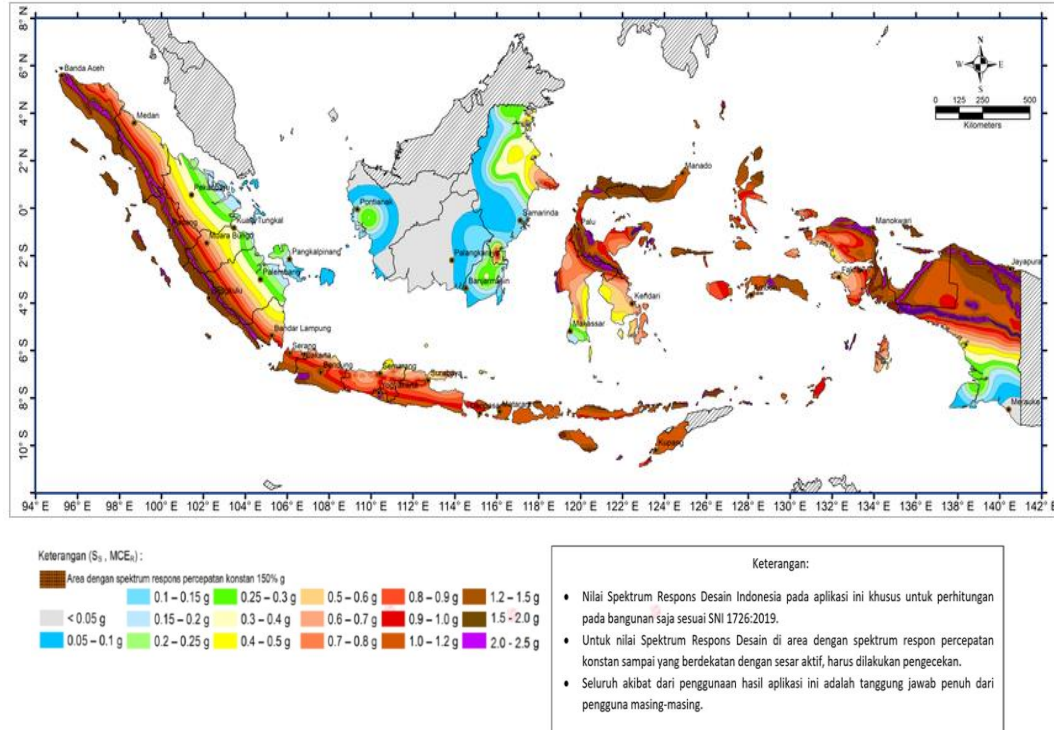
Gambar 3. 3 Akselerasi respon spektrum, SS
