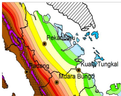
Gambar 5. 8 Akselerasi respon spektrum, SS Sumber : (PUPR, 2021)
