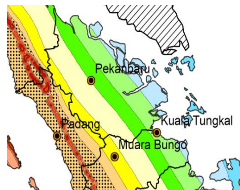
Gambar 5. 9 Akselerasi respon spektrum, S1 Sumber : (PUPR, 2021)
