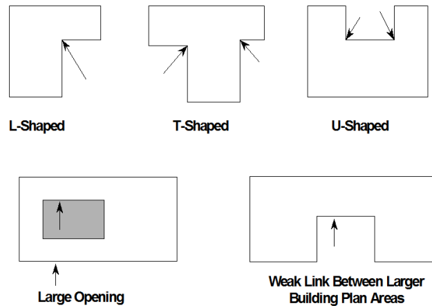
Gambar 3. 11 Ketidak teraturan secara datar
