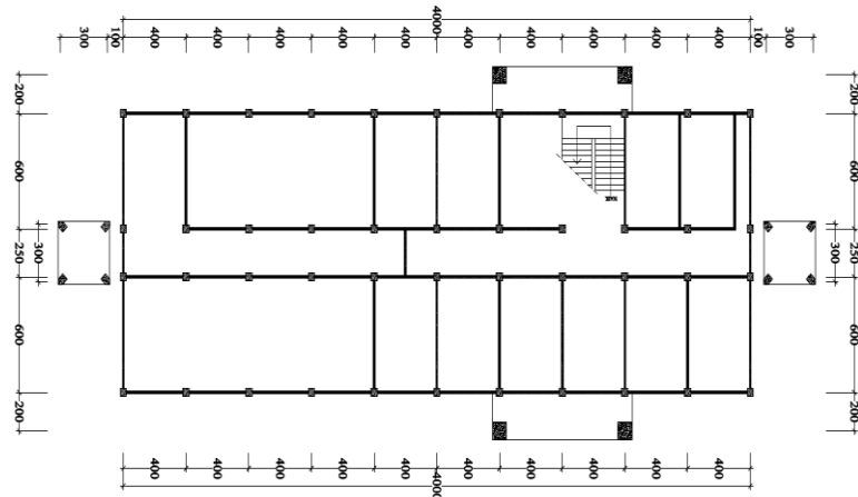
Gambar 5. 15 Denah Lantai 1 Kantor Tata Pemerintahan, Hukum, dan Politik Kampar
