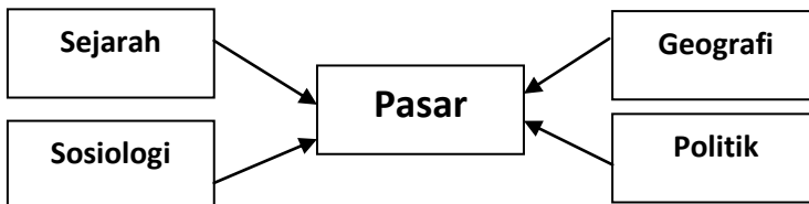
Gambar 2: Pendekatan Monodisiplin
